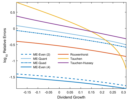
(d) \rho = 0.95, \gamma = 1.3, N = 21.
